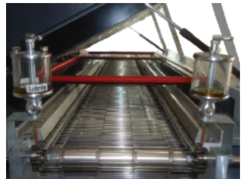
Edge Pin Above Mesh Conveyor
